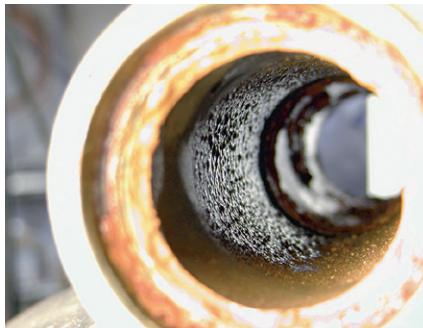
Samma galvaniserade kallvattenrör ca 16 månader efter installationen av Bauer
