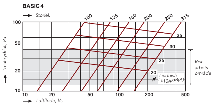
BASIC 4 (med Irisspjäll)
